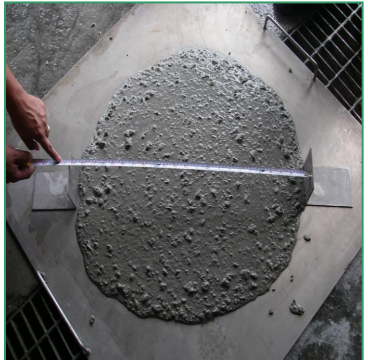
SCC R1 坍流度 65cm~75cm 通過 50 公分圓周時間 6.8 秒 90 分鐘後坍流度 69cm
